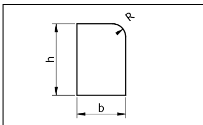
Rys. 1. Wymiarowanie krawężników
